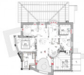
2 ЭТАЖ
